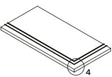
* step tread "L" corner inox nez de marche "L" angle inox ecke stufenplatte "L" inox degrau "L" canto inox 30x60 NR . TC MP-6650 30x120 NR . TC MP-6710
