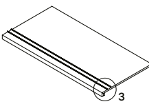
step tread "L" inox nez de marche "L" inox stufenplatte "L" inox degrau "L" inox 30x60 NR MP-6580 30x90 NR . MP-6640 30x120 NR MP-6670
