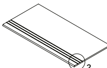
step tread grooved nez de marche creusé stufenplatte mit rillen degrau sulcado 30x60 NR MP-6240 30x90 NR . ASR MP-6430 30x120 NR MP-6445
