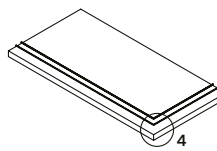
* step tread "L" corner inox nez de marche "L" angle inox ecke stufenplatte "L" inox degrau "L" canto inox 30x60 NR MP-6650 30x90 NR . MP-6690 30x120 NR MP-6710
