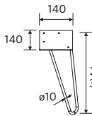
CONJUNTO DE 2 PÉS UNIIQ 230 / 330
