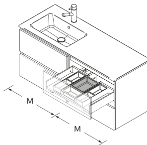
BANDEJA SIFÃO
