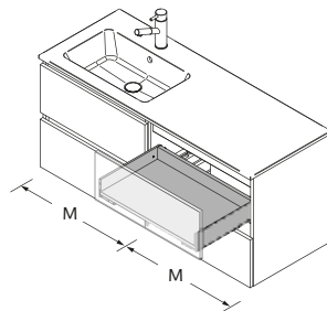
GAVETA METÁLICA SEM ABERTURA PARA SIFÃO
