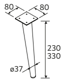
CONJUNTO DE 2 PÉS DANNA 230 / 330
