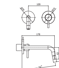
LIG BOX105-104-106CR70 Miscelatore incasso con bocca erogazione a muro 178 mm / 123 mm / 248 mm Corpo incasso da ordinare separatamente Concealed wash basin mixer with wall spout 178 mm / 123mm / 248 mm Built_in box o be ordered seprately
