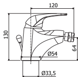
DU 131-135CR Miscelatore bidet con/senza scarico Bidet mixer with/without pop up waste
