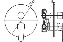
SY 015CR Miscelatore incasso doccia con deviatore corpo incasso incluso Concealed shower mixer with diverter concealed body included
