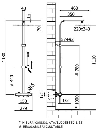
ZCOL 665CR CITY Colonna doccia con miscelatore termostatico Shower column with thermostatic mixer
