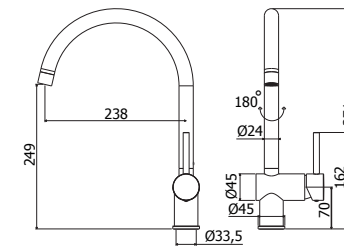
LIG 280CR Miscelatore lavello monoforo con canna orientabile One-hole sink mixer with swivelling spout
