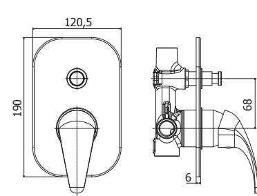
ND 015CR Miscelatore incasso doccia con deviatore corpo incasso incluso Concealed shower mixer with diverter concealed body included
