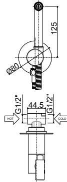
ZDUP 128CR TWEET LOCK Set bidet incasso con miscelatore e chiusura di sicurezza, doccia 2 getti Concealed bidet set with mixer and safety clo- sing system, 2 spray hand shower
