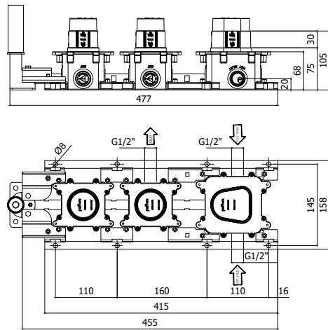
MDBOX 000 Set incasso per miscelatore termostatico doccia/va- sca (2 funzioni) - Installazione solo orizzontale Concealed set for thermostatic shower/bath mixer (2 functions) - Horizontal installation only
