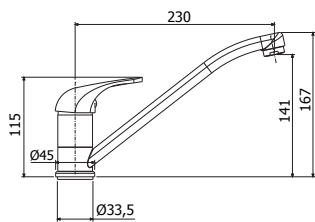
APM3 182CR Miscelatore lavello monoforo con canna tubo orientabile One-hole sink mixer with tube swivelling spout
