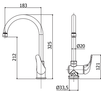
APM3 180CR Miscelatore lavello monoforo con canna tubo orientabile One-hole sink mixer with tube swivelling spout
