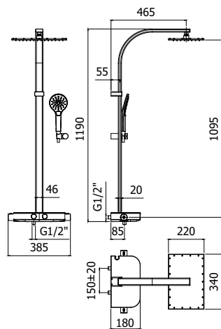
ZCOL 668CRAG MOBY Colonna doccia con miscelatore termostatico Shower column with thermostatic mixer
