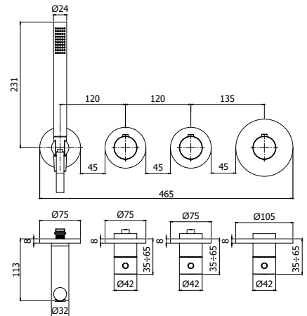
MDE 000 Set esterno per miscelatore termostatico incasso doc- cia/vasca (2 funzioni) - Installazione solo orizzontale External set for concealed thermostatic shower/bath mixer (2 functions) - Horizontal installation only
