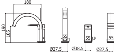
LES 040CR-041CR Batteria miscelatore bordo vasca con doccia estraibile, con/senza bocca erogazione Deck-mounted bath mixer with pull out hand-shower, with/without spout
