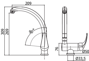
ND 189CR Miscelatore lavello laterale canna reclinabile sotto finestra One-hole sink mixer below window
