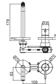
BI 105-104-106CR70 Miscelatore incasso con bocca erogazione a muro 178 mm / 123 mm / 248 mm corpo incasso incluso Concealed wash basin mixer with wall spout 178 mm / 123 mm / 248 mm concealed body included
