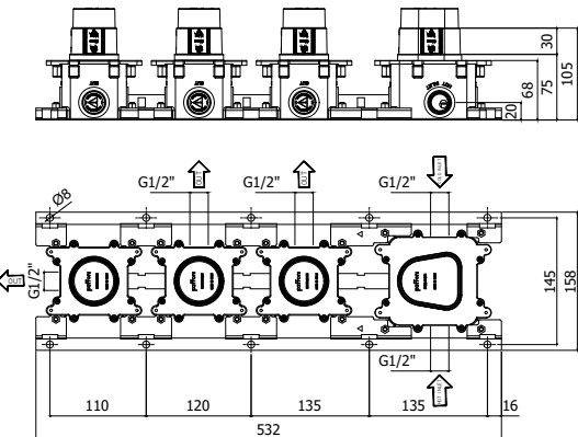
MDBOX 019 Set incasso per miscelatore termostatico doccia/va- sca (3 funzioni) - Installazione orizzontale o verticale Concealed set for thermostatic shower/bath mixer (3 functions) - Horizontal or vertical installation
