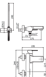
RIN 022-023-026 CR Miscelatore vasca/doccia con/senza set doccia, con supporto a muro fisso ABS Bath/shower mixer with/without shower set, with ABS fixed wall bracket
