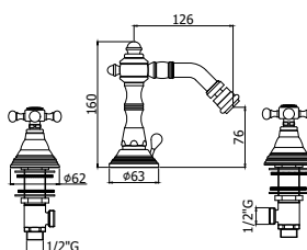
FBLV 118-119 CR Batteria bidet con bocca erogazione, con/senza scarico Three-hole bidet mixer with spout, with/without pop up waste
