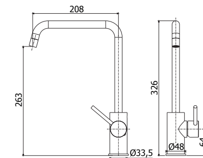
LIG 980CR Miscelatore lavello monoforo con canna orientabile One-hole sink mixer with swivelling spout
