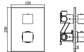
LEQ 519CR Miscelatore termostatico incasso doccia con deviatore 3 uscite corpo incasso incluso Concealed thermostatic shower mixer with diverter 3 outlets concealed body included
