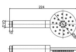
ZDOC 133AC INOX Doccia Inox (monogetto) in acciaio Ø90mm Inox (single-spray) steel hand- shower Ø90mm
