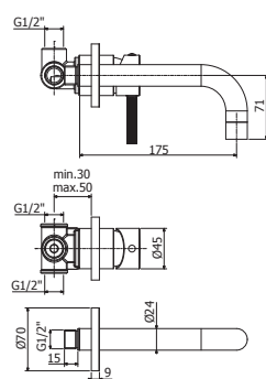
FOX 006 - 007 CR 70 Miscelatore vasca/doccia incasso completo di deviatore, bocca 175 - 245mm e set doccia corpo incasso incluso Concealed bath/shower mixer complete with diverter, spout and shower kit concealed body included
