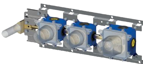
MDBOX 000 Set incasso per miscelatore termostatico doccia/va- sca (2 funzioni) - Installazione solo orizzontale Concealed set for thermostatic shower/bath mixer (2 functions) - Horizontal installation only
