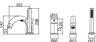
JL 047 - JL048 CR Miscelatore bordo vasca con doccia estraibile, con/senza bocca erogazione Deck mounted bath mixer with pull out hand-shower, with/without spout
