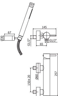
BI 168L-168DL-168RL Miscelatore doccia attacco 1/2" con/ senza set doccia, rovesciato senza set doccia Shower mixer 1/2" connection with/ without shower kit, overturned without shower kit
