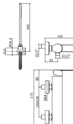
TA 168-168DCR Miscelatore doccia con/senza set doccia Shower mixer with/without shower set
