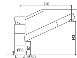
BI 182CR Miscelatore lavello monoforo con canna orientabile One-hole sink mixer with swivelling spout
