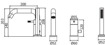
JL 045CR Miscelatore bordo vasca con doccia estraibile, con/senza bocca erogazione Deck mounted bath mixer with pull out hand-shower, with/without spout
