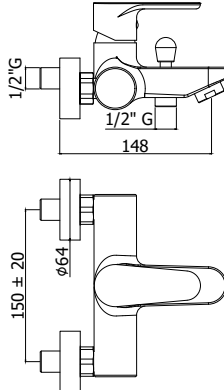
GR 022-023CR Miscelatore vasca/doccia con/ senza set doccia Bath/shower mixer with/ without shower set
