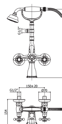
FBLV 022-023CR Gruppo vasca lusso con set doccia - Flessibile 1000 e 1500 mm Bath shower mixer lux-model with shower set - Flexible hose 1000 and 1500 mm
