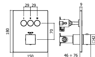
CPT 519CR Set esterno termostatico incasso doccia (3 funzioni) con deviatore a pulsante On/Off External set for concealed thermostatic shower mixer (3 functions) with push diverter On/Off
