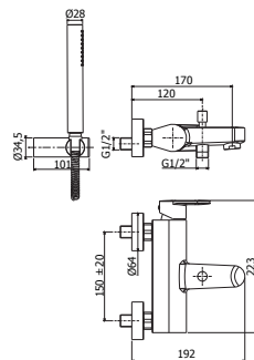
CA 022-023-026CR Miscelatore vasca/doccia con/senza set doccia, con supporto fisso in ABS Bath/shower mixer with/without shower set, with ABS fixed bracket
