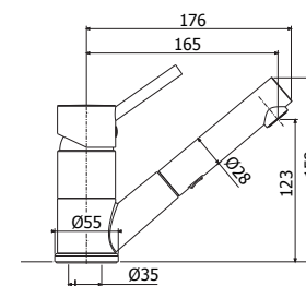
BI 183CR Miscelatore lavello monoforo con doccia estraibile (2 getti) e canna orientabile One-hole sink mixer with pull out hand-shower (two-spray) and swivelling spout
