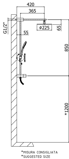
ZCOL 687CR UP Colonna doccia senza miscelatore, con presa acqua superiore Shower column without mixer, with upside water inlet
