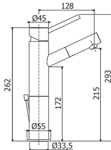
BI 071CR93 Miscelatore lavabo con prolunga 100 mm Wash basin mixer with extension 100 mm
