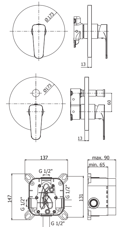
PBOX 001 Set incasso universale per miscelatori doccia Universal Concealed Box for mixers
