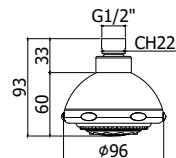
ZSOF 030CR ISCHIA Soffione "Ischia" in ABS, anticalcare Ø 96 mm "Ischia" ABS shower head, antiscala system Ø 96 mm
