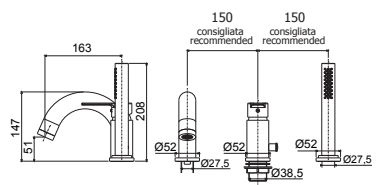
RED 040L-041LCR Batteria miscelatore bordo vasca con doccia estraibile, con/senza bocca erogazione Deck-mounted bath mixer with pull out hand-shower, with/without spout
