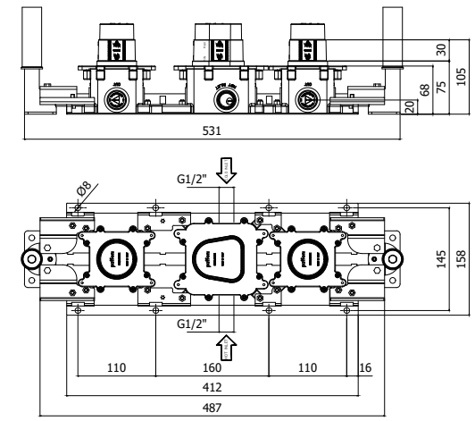
MDBOX 001 Set incasso per miscelatore termostatico doccia/va- sca (2 funzioni) - Installazione solo orizzontale Concealed set for thermostatic shower/bath mixer (2 functions) - Horizontal installation only
