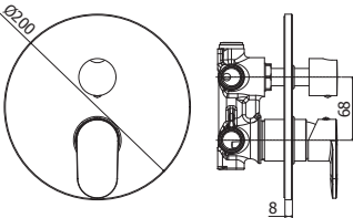
CA 018-019CR Miscelatore incasso doccia con deviatore 2 uscite/3 uscite corpo incasso incluso Concealed shower mixer with diverter 2 outlets/3 outlets concealed body included
