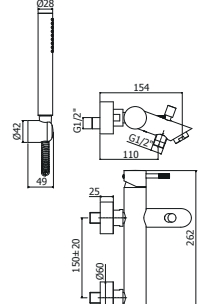
JL 026CR Miscelatore vasca/doccia con set doccia e supporto a muro fisso in ABS Bath/shower mixer with shower set and ABS fixed wall bracket
