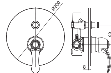
FA 015CR Miscelatore incasso doccia con deviatore corpo incasso incluso Concealed shower mixer with diverter concealed body included
