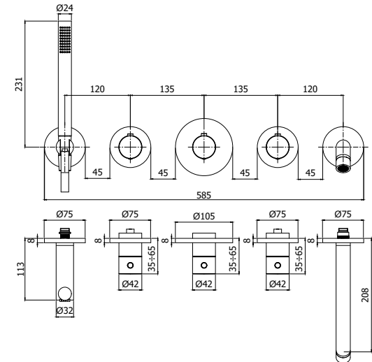
MDE 001 Set esterno per miscelatore termostatico incasso doc- cia/vasca (2 funzioni) - Installazione solo orizzontale External set for concealed thermostatic shower/bath mixer (2 functions) - Horizontal installation only
