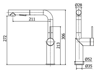
INOX 285AC Miscelatore lavello monoforo con canna orientabile con doccia estraibile Dualjet One-hole sink mixer with swivelling spout with Dualjet pull out hand-shower
