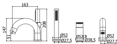
CA 040-041CR Batteria miscelatore bordo vasca con doccia estraibile, con/senza bocca erogazione Deck mounted bath mixer with pull-out hand-shower, with/without spout
