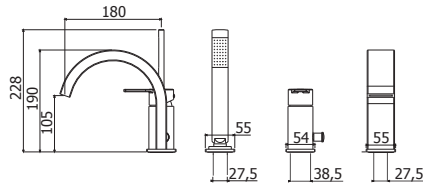
RIN 040L-041LCR Batteria miscelatore bordo vasca con doccia estraibile, con/senza bocca erogazione Deck-mounted bath mixer with pull out hand-shower, with/without spout
