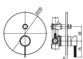
FOX 015CR Miscelatore incasso doccia con deviatore corpo incasso incluso Concealed shower mixer with diverter concealed body included
