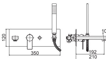
TA 001CR Miscelatore incasso vasca/doccia completo di deviatore, bocca e set doccia corpo incasso incluso Concealed bath/shower mixer with diverter, spout and shower kit concealed body included
