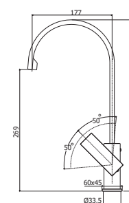
EL 880CR Miscelatore lavello monoforo con canna orientabile One-hole sink mixer with swivelling spout
