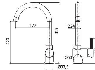
FOX 180CR Miscelatore lavello monoforo con canna orientabile One-hole sink mixer with swivelling spout
