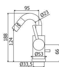
BI 138-137CR Miscelatore bidet con canna orientabile con/ senza scarico Bidet mixer with swivelling spout with/ without pop up waste
