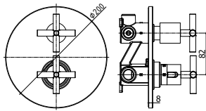
QTV 018CR Miscelatore termostatico incasso doccia con deviatore 2 uscite corpo incasso incluso Concealed thermostatic shower mixer with diverter 2 outlets concealed body included
