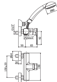
DU 168-168DCR Miscelatore doccia con/senza set doccia Shower mixer with/without shower set
