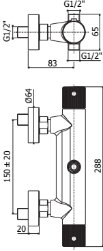
JOQ 169CR Miscelatore termostatico doccia (2 uscite) con attacco 1/2" x 1/2" con deviatore Thermostatic shower mixer (2 outlets) 1/2" x 1/2" connection with diverter
