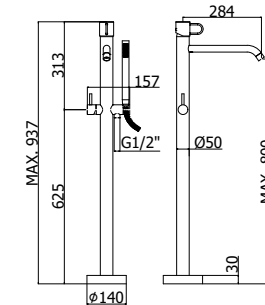
JKBOX 032CR Miscelatore vasca/doccia a pavimento Free-standing bath/shower mixer
