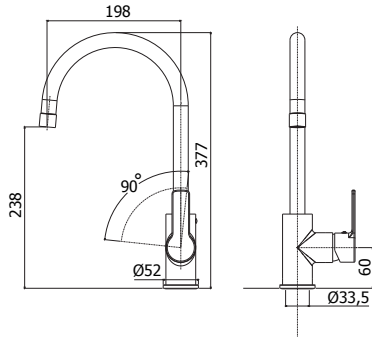
RED 180CR Miscelatore lavello monoforo con canna orientabile One-hole sink mixer with swivelling spout
