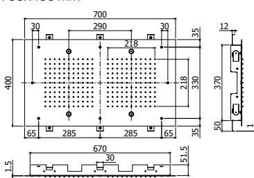
ZSOF 131CR MEMPHIS Soffione ad incasso in metallo, anticalcare, con NEBULIZZATORE - 700x400 mm Concealed ceiling metal shower head, antiscaling system, with NEBULIZER JETS - 700x400 mm
