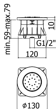
ZSOF 120CR Soffione tondo in ABS, anticalcare, con getto orientabile - Ø130 mm Round ABS body jet, antiscaling system, with swivelling spray - Ø130 mm
