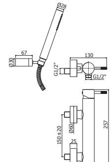
JL 168-168D-168R CR Miscelatore doccia esterno attacco 1/2" con/senza set doccia, e rovesciato senza set doccia Shower mixer 1/2" connection with/without shower set, and mixer overturned without shower set
