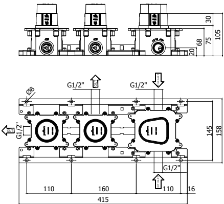
MDBOX 018 Set incasso per miscelatore termostatico doccia/va- sca (2 funzioni) - Installazione orizzontale o verticale Concealed set for thermostatic shower/bath mixer (2 functions) - Horizontal or vertical installation
