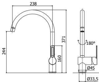
RIN 180CR Miscelatore lavello monoforo alto con canna orientabile Tall one-hole sink mixer with swivelling spout
