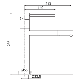
BI 188CR Miscelatore lavello monoforo alto con canna orientabile Tall one-hole sink mixer with swivelling spout
