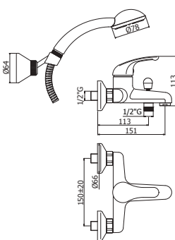
APM3 022-023CR Miscelatore vasca con/ senza set doccia Bath/shower mixer with/ without shower set
