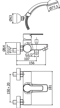
ND 022-023-026CR Miscelatore vasca con/ senza set doccia, con supporto a muro fisso ABS Bath/shower mixer with/ without shower set, with ABS fixed wall bracket
