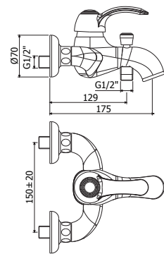
FA 022-024CR Miscelatore vasca/doccia con/ senza set doccia Bath/shower mixer with/ without shower set
