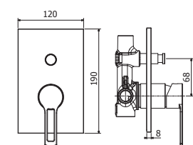
RIN 015CR Miscelatore incasso doccia con deviatore corpo incasso incluso Concealed shower mixer with diverter concealed body included
