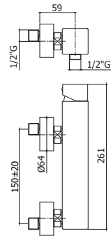
LEC 168-168D-168R CR Miscelatore doccia con/senza set doccia, rovesciato Shower mixer with/without shower set, overturned
