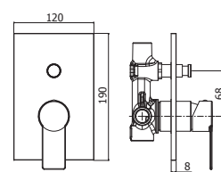
TA 015CR Miscelatore incasso doccia con deviatore corpo incasso incluso Concealed shower mixer with diverter concealed body included
