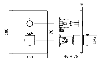
CPT 513CR Set esterno termostatico incasso doccia (1 funzione) con deviatore a pulsante On/Off External set for concealed thermostatic shower mixer (1 function) with push diverter On/Off
