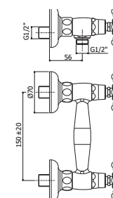
FBLV 168-168DCR Gruppo doccia con/senza set doccia Wall shower mixer with/without shower set
