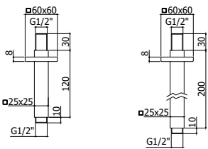
ZSOF 118-119CR Braccio doccia a soffitto - 25x25 mm - L.120/ 200 mm Ceiling shower arm - 25x25 mm - L.120/ 200 mm
