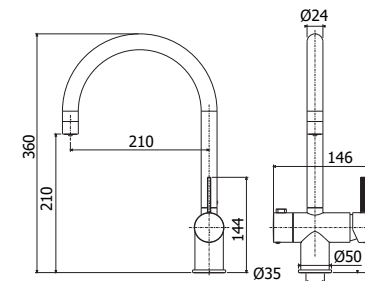
FOX 192CR - DRINKING SYSTEM Miscelatore lavello monoforo con canna orientabile e 3° ingresso per acqua depurata e passaggio delle acque separato One-hole sink mixer with 3rd swivelling spout inlet for purified water and double water passages
