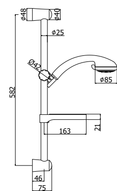
ZSAL 090CR2 CRETA DUE Saliscendi Creta due con doccia (3 getti) in ABS Creta due sliding rail with (3-spray functions) ABS hand-shower
