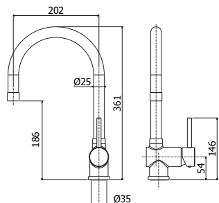
SK 185CR Miscelatore lavello con canna orientabile e doccetta estraibile One-hole sink mixer with swivelling spout and pull out spray
