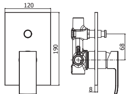
EL 015CR Miscelatore incasso doccia con deviatore corpo incasso incluso Concealed shower mixer with diverter concealed body included
