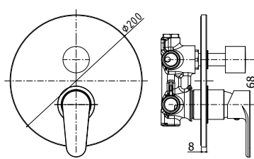
GR 018-019CR Miscelatore incasso doccia con deviatore 2 uscite/3 uscite corpo incasso incluso Concealed shower mixer with diverter 2 outlets/3 outlets concealed body included
