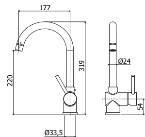
SK 180CR Miscelatore lavello monoforo con canna orientabile One-hole sink mixer with swivelling spout
