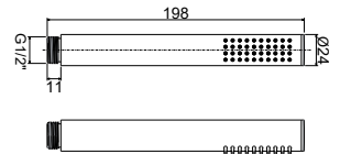
ZDOC 132AC INOX Doccia Minimal (monogetto) in acciaio Minimal (single-spray) steel hand-shower
