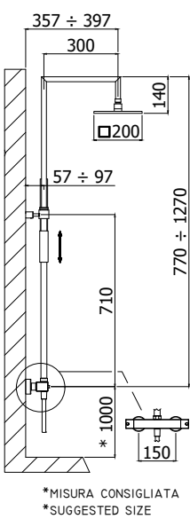
ZCOL 655CR SYNCRO TOP Colonna doccia con miscelatore termostatico Shower column with thermostatic mixer
