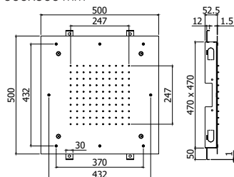
ZSOF 129CR CLEVELAND Soffione ad incasso in metallo, anticalcare, con NEBULIZZATORE - 500x500 mm Concealed ceiling metal shower head, antiscaling system, with NEBULIZER JETS - 500x500 mm
