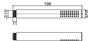
ZDOC 132AC INOX Doccia Inox (monogetto) in acciaio Inox (single-spray) steel hand- shower
