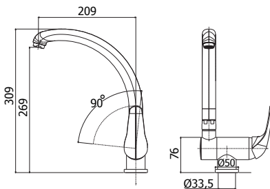
DU 189CR Miscelatore lavello laterale canna reclinabile sotto finestra One-hole sink mixer below window
