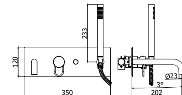
JK 001CR Miscelatore incasso vasca/doccia completo di deviatore, bocca e set doccia corpo incasso incluso Concealed bath/shower mixer with diverter, spout and shower kit concealed body included
