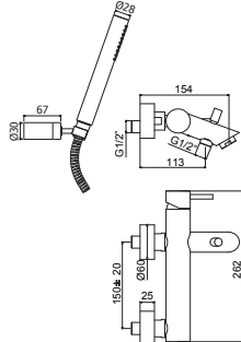
LIG 022-023-026CR Miscelatore vasca/doccia con/senza set doccia, con supporto a muro fisso ABS Bath/shower mixer with/without shower set, with ABS fixed wall bracket
