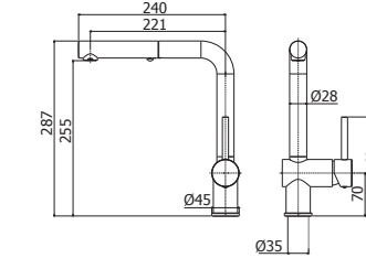
LIG 285CR-MET Miscelatore lavello monoforo con canna orientabile con doccia estraibile Dualjet One-hole sink mixer with swivelling spout with Dualjet pull out hand-shower
