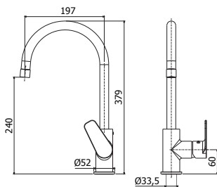
LM 180CR Miscelatore lavello monoforo con canna a tubo orientabile One-hole sink mixer with tube swivelling spout
