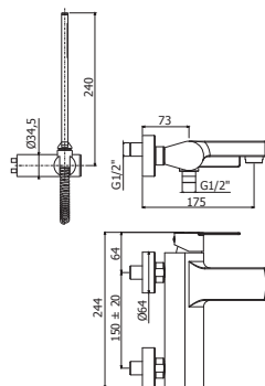
TA 022-023-026 CR Miscelatore vasca doccia con/senza set doccia, con supporto fisso Bath/shower mixer with/without shower set, with fixed bracket
