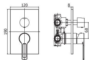
RIN 018-019CR Miscelatore incasso doccia con deviatore 2 uscite/3 uscite corpo incasso incluso Concealed shower mixer with diverter 2 outlets/3 outlets concealed body included
