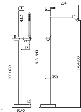
JLBOX 032CR Miscelatore vasca/doccia a pavimento Corpo incasso da ordinare separatamente Free-standing bath/shower mixer Built_in box o be ordered separately
