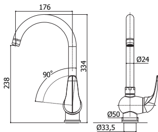
DU 180CR Miscelatore lavello monoforo con canna tubo orientabile One-hole sink mixer with tube swivelling spout
