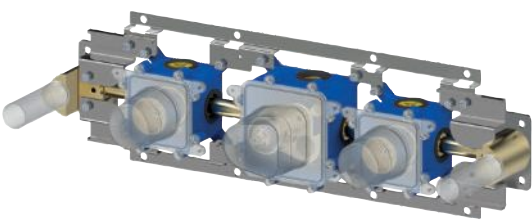
MDBOX 001 Set incasso per miscelatore termostatico doccia/va- sca (2 funzioni) - Installazione solo orizzontale Concealed set for thermostatic shower/bath mixer (2 functions) - Horizontal installation only
