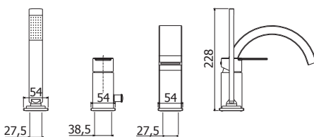
TA 040-041CR Batteria miscelatore bordo vasca con doccia estraibile, con/senza bocca estribile Deck mounted bath mixer with pull out hand-shower, with/without spout
