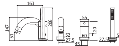
BI 047-048CR MAX FLOW Miscelatore bordo vasca con doccia estraibile, con/senza bocca erogazione Deck mounted bath mixer with pull out hand-shower, with/without spout
