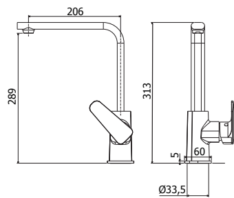
SY 180CR Miscelatore lavello monoforo con canna piatta orientabile One-hole sink mixer with flat swivelling spout
