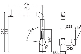
RIN 285CR - RIN 185CR Miscelatore lavello monoforo con doccia ABS estraibile (2 getti) - (RIN185 monogetto) e canna orientabile One-hole sink mixer with pull-out ABS handshower (two-spray) - (RIN185 single-spray) and swivelling spout
