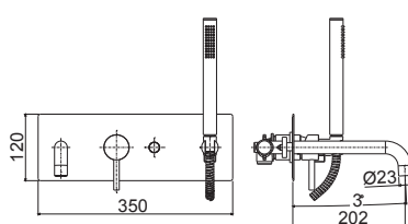
LIG 001CR Miscelatore incasso vasca/doccia completo di deviatore, bocca e set doccia corpo incasso incluso Concealed bath/shower mixer with diverter, spout and shower kit concealed body included
