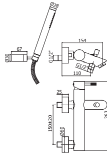
JL 022-023CR Miscelatore vasca/doccia con/senza set doccia Bath/shower mixer with/without shower set
