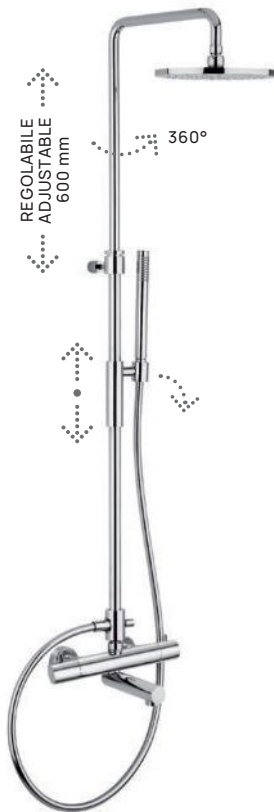
ZCOL 721LIQCR BIRILLO Colonna doccia con miscelatore termostatico vasca Shower column with thermostatic bath/ shower mixer
