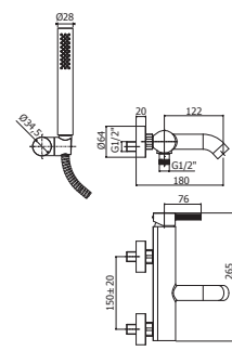
FOX 022-023CR Miscelatore vasca/doccia con/ senza set doccia Bath/shower mixer with/ without shower set
