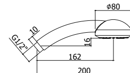
ZDOC 081CR TRIESTE BIS Doccia Trieste bis (monogetto) in ABS Trieste bis (single-spray) ABS hand-shower
