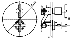
QTV 019CR Miscelatore termostatico incasso doccia con deviatore 3 uscite corpo incasso incluso Concealed thermostatic shower mixer with diverter 3 outlets concealed body included
