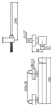
EL 168-168DCR-168R Miscelatore doccia con/senza set doccia, rovesciato Shower mixer with/without shower set, overturned
