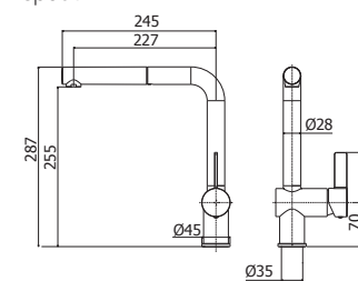
RO 185CR Miscelatore lavello monoforo con doccia estraibile (monogetto) e canna orientabile One-hole sink mixer with pull-out hand-shower (single-spray) and swivelling spout
