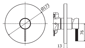
FOX BOX010CR Set esterno miscelatore incasso doccia senza deviatore External set for concealed shower mixer without diverter
