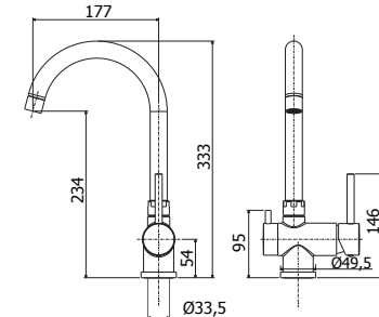
SK 190CR 3 VIE Miscelatore lavello monoforo con canna orientabile e 3° ingresso per acqua depurata One-hole sink mixer with swivelling spout 3rd inlet for purified water
