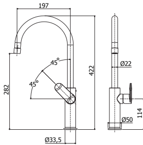
CA 180CR Miscelatore lavello monoforo alto con canna orientabile Tall one-hole sink mixer with swivelling spout
