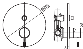
JL 015CR Miscelatore incasso doccia (2 uscite) con deviatore a pulsante corpo incasso incluso Concealed shower mixer (2 outlets) with push diverter concealed body included
