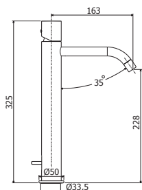
LIGX 081-085CR Miscelatore lavabo prolungato con leva cilindro Tall wash basin mixer with cilindro handle
