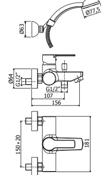
RED 022-023-024-026CR Miscelatore vasca/doccia con/senza set doccia, con supporto fisso in ABS, con supporto snodato Stick Bath/shower mixer with/without shower set, with ABS fixed bracket, with Stick wall bracket
