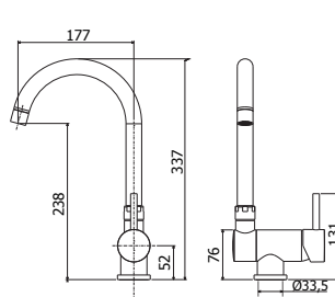
SK 189CR Miscelatore lavello monoforo con canna reclinabile sotto finestra One-hole sink mixer with below windows
