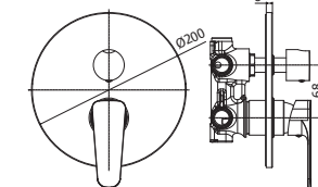
SY 018-019CR Miscelatore incasso doccia con deviatore 2 uscite/3 uscite corpo incasso incluso Concealed shower mixer with diverter 2 outlets/3 outlets concealed body included
