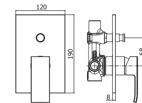
LES 015CR Miscelatore incasso doccia con deviatore corpo incasso incluso Concealed shower mixer with diverter concealed body included
