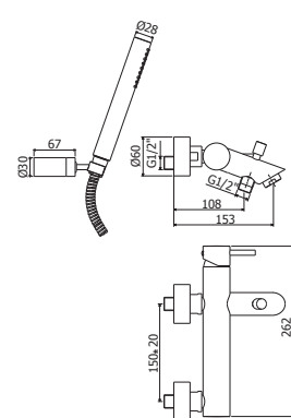
BI 022L-023L-026LCR Miscelatore vasca/doccia con/ senza set doccia, con supporto a muro fisso ABS Bath/shower mixer with/ without shower set, with ABS fixed wall bracket
