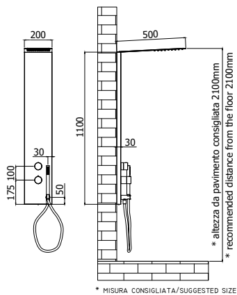
ZCOL 673CR GAMMA Colonna doccia con miscelatore termostatico Shower column with thermostatic mixer
