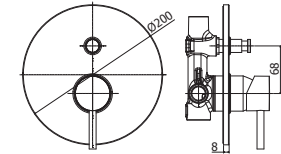
BI 015CR35 Miscelatore incasso doccia (2 uscite) con deviatore a pulsante corpo incasso incluso Concealed shower mixer (2 outlets) with push diverter concealed body included
