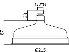
ZSOF 046CR BELINDA Soffione "Belinda" in metallo, design Retrò Ø 215 mm "Belinda" metal shower head, Retrò design Ø 215 mm
