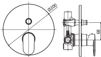
CA 015CR Miscelatore incasso doccia con deviatore corpo incasso incluso Concealed shower mixer with diverter concealed body included
