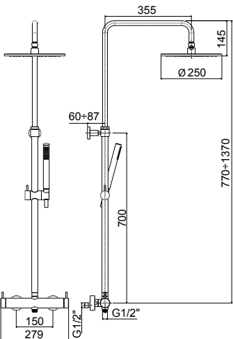
ZCOL 504AC INOX TECH Colonna doccia con miscelatore INOX169AC Shower column with mixer INOX169AC
