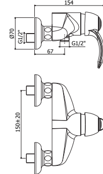
FA 168-168DCR Miscelatore doccia con/ senza set doccia Shower mixer with/ without shower set
