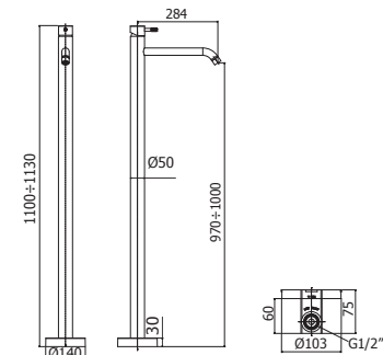
JLBOX 031CR Miscelatore lavabo a pavimento Corpo incasso da ordinare separatamente Free-standing basin mixer Built_in box o be ordered separately
