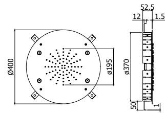
ZSOF 130CR FILADELFIA Soffione ad incasso in metallo, anticalcare, con NEBULIZZATORE - Ø 400 mm Concealed ceiling metal shower head, anti- scale system, with NEBULIZER JETS - Ø 400 mm
