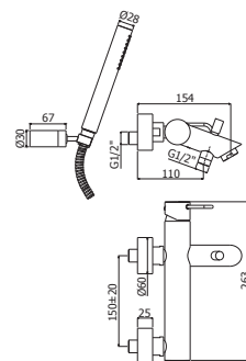
JK 022-023-026CR Miscelatore vasca/doccia con/senza set doccia, con supporto a muro fisso ABS Bath/shower mixer with/without shower set, with ABS fixed wall bracket
