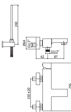
EL 022-023-026CR Miscelatore vasca doccia con/senza set doccia, con supporto a muro fisso ABS Bath/shower mixer with/without shower set, with ABS fixed wall bracket
