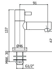
MI 090CR Rubinetto lavabo solo acqua fredda Basin tap cold water only
