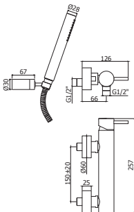
LIG 168-168D - 168R CR Miscelatore doccia esterno attacco 1/2" con/senza set doccia e rovesciato senza set doccia Shower mixer 1/2" connection with/wi- thout shower set and overturned without shower set
