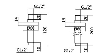
ZSOF 064-065CR Braccio doccia a soffitto - Ø 24 mm - L.120/200 mm Ceiling shower arm - Ø 24 mm - L.120/200 mm
