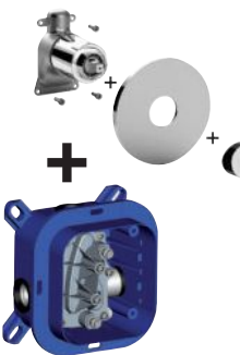
BI BOX010CR Set esterno miscelatore incasso doccia senza deviatore External set for concealed shower mixer without diverter
