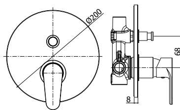
GR 015CR Miscelatore incasso doccia con deviatore corpo incasso incluso Concealed shower mixer with diverter concealed body included
