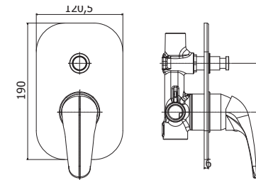
DU 015CR Miscelatore incasso doccia con deviatore corpo incasso incluso Concealed shower mixer with diverter concealed body included
