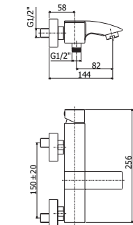
LEC 022-023-026CR Miscelatore vasca doccia con/senza set doccia, con supporto fisso Bath/shower mixer with/without shower set, with wall fixed bracket
