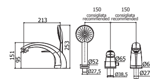
DU 040-041CR Batteria miscelatore bordo vasca con doccia estraibile, con/senza bocca erogazione Deck mounted bath mixer with pull out hand-shower, with/ without spout
