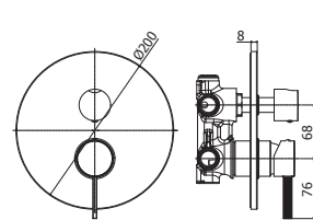
FOX 018-019CR Miscelatore incasso doccia con deviatore 2 uscite/3 uscite corpo incasso incluso Concealed shower mixer with diverter 2 outlets/3 outlets concealed body included
