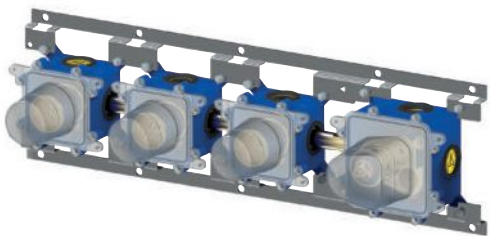
MDBOX 019 Set incasso per miscelatore termostatico doccia/va- sca (3 funzioni) - Installazione orizzontale o verticale Concealed set for thermostatic shower/bath mixer (3 functions) - Horizontal or vertical installation
