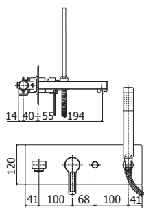
RIN 001CR Miscelatore vasca/doccia incasso completo di deviatore, bocca e set doccia corpo incasso incluso Concealed bath/shower mixer complete with diverter, spout and shower kit concealed body included
