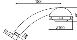
ZDOC 045CR ISCHIA Doccia Ischia (3 getti) in ABS Ø100 Ischia (3-spray functions) ABS hand-shower Ø100
