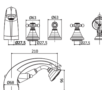
FBLV 040-041CR Batteria bordo vasca 5 fori con doccia estraibile, con/senza bocca erogazione Five-hole bath mixer deck-mounted with hand-shower, with/without spout
