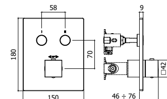
CPT 518CR Set esterno termostatico incasso doccia (2 funzioni) con deviatore a pulsante On/Off External set for concealed thermostatic shower mixer (2 functions) with push diverter On/Off
