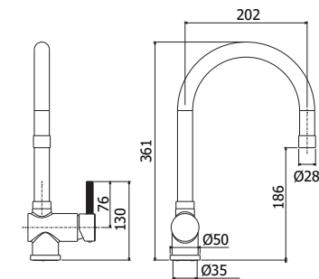
FOX 185CR Miscelatore lavello con canna orientabile e doccetta estraibile One-hole sink mixer with swivelling spout and pull out spray
