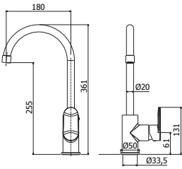
CA 181CR Miscelatore lavello monoforo con canna orientabile One-hole sink mixer with swivelling spout
