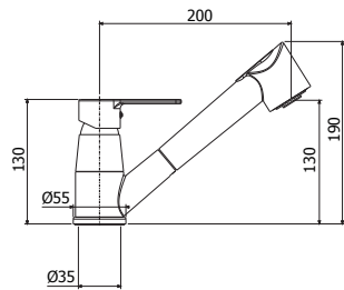
RED 183CR Miscelatore lavello con doccia estraibile (2 getti) e canna orientabile One-hole sink mixer with pull-out hand-shower and swivelling spout
