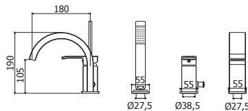
EL 040-041CR Batteria miscelatore bordo vasca con doccia estraibile, con/senza bocca erogazione Deck mounted bath mixer with pull out hand-shower, with/without spout
