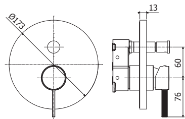
FOX BOX015CR Set esterno miscelatore incasso doccia con deviatore External set for concealed shower mixer with diverter
