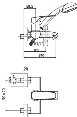
LM 022-023-026 CR Miscelatore vasca/doccia con/senza set doccia, con supporto a muro fisso ABS Bath/shower mixer with/without shower set, with ABS fixed wall bracket
