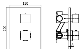
LEQ 518CR Miscelatore termostatico incasso doccia con deviatore 2 uscite corpo incasso incluso Concealed thermostatic shower mixer with diverter 2 outlets concealed body included
