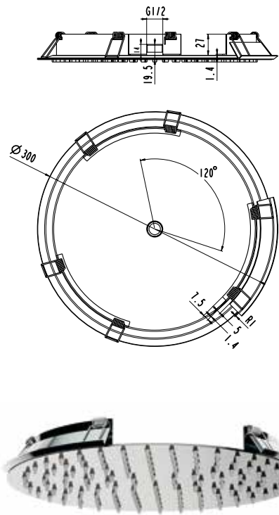
ROCIADOR REDONDO EMPOTRADO Ø30 cm Material: Acero Inox SS304
