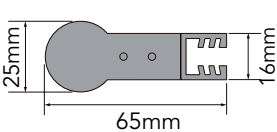
Perfil Profile
